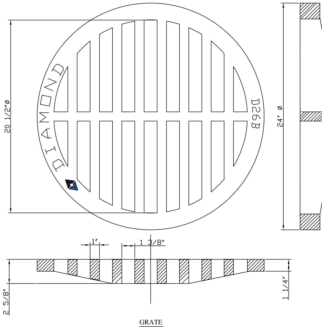
D26B:-24" Cast Iron Grate for D26B Frame
